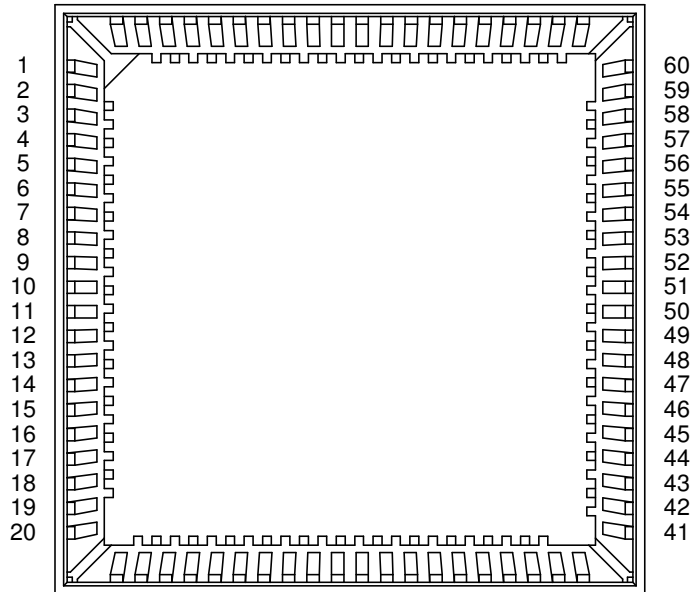
M-QFN80 80L
