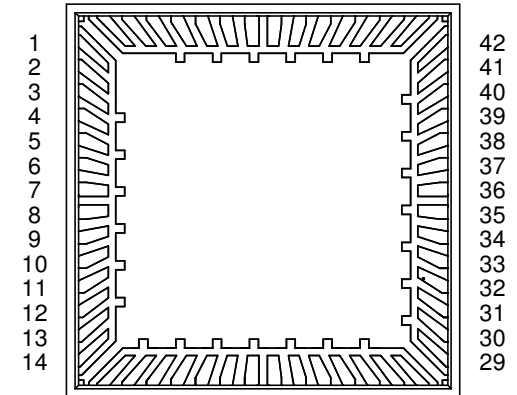
M-QFN56 56L
